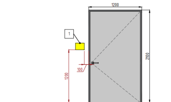
Тактильная табличка перед дверью в помещение
