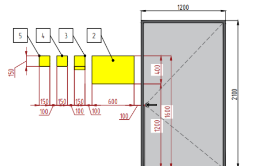
Тактильная табличка перед дверью в помещение
